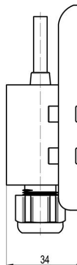
Typ 31141 mit externem Temperaturfühler und Sonnenschutzdach
